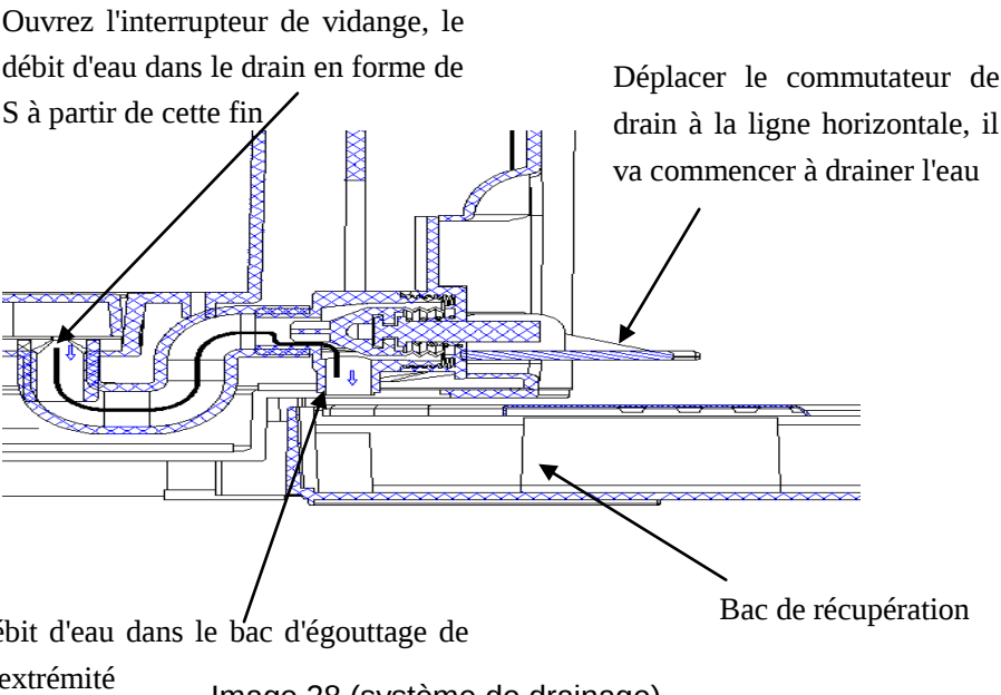
Image 28 (système de drainage)
