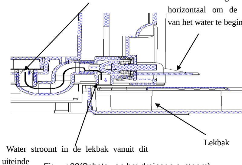
Figuur 28(Schets van het drainage systeem)
