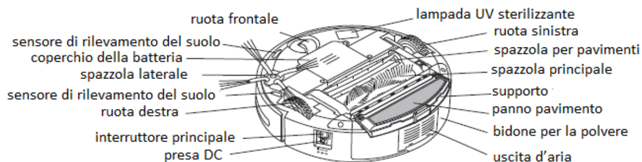
Parte inferiore del corpo macchina
